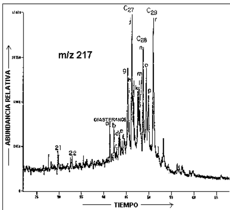
Distribución de biomarcadores esteranos m/z 217 de la impregnación de petróleo Imp-1 (Tomado de: Del Olio, 1993)
