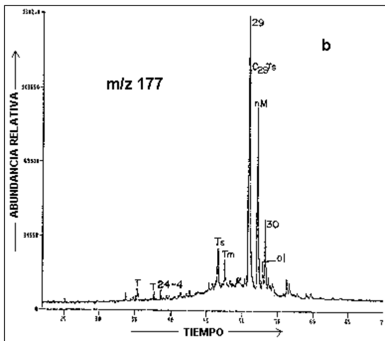
Distribución de biomarcadores terpanos m/z 191(a) y m/z 177(b) de la impregnación de petróleo Imp-1 (Tomado de: Del Olio, 1993)
