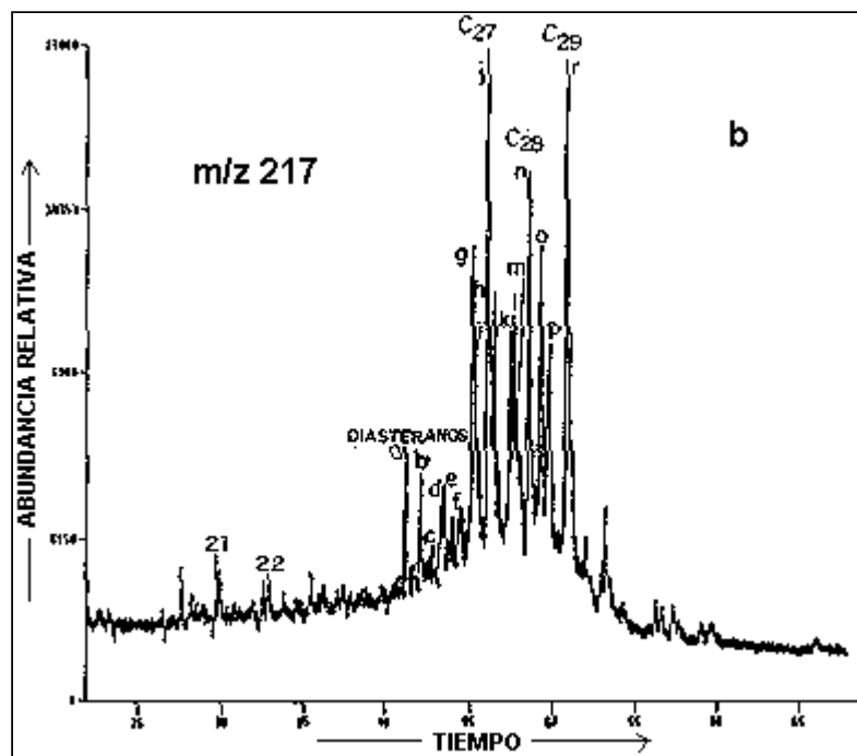
Comparación de distribución de esteranos de (a) ATP-30 y (b) Imp-1 (Tomado de: Del Olio, 1993)
