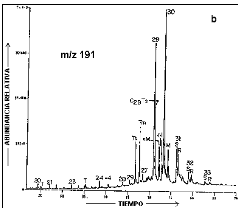
Comparación de distribución de terpanos de (a) ATP-32 y (b) Imp-1 (Tomado de: Del Olio, 1993)
